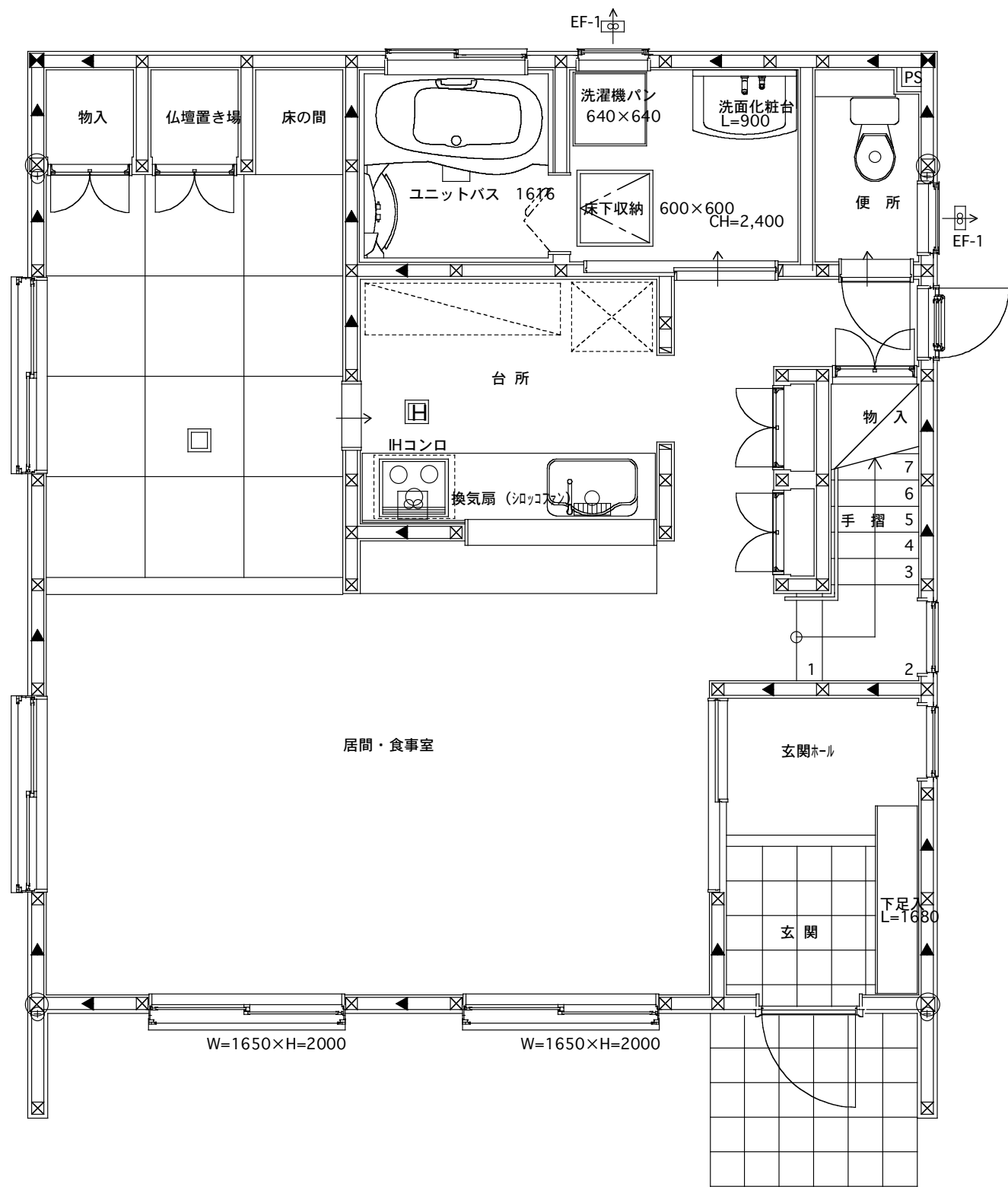
1階平面図
