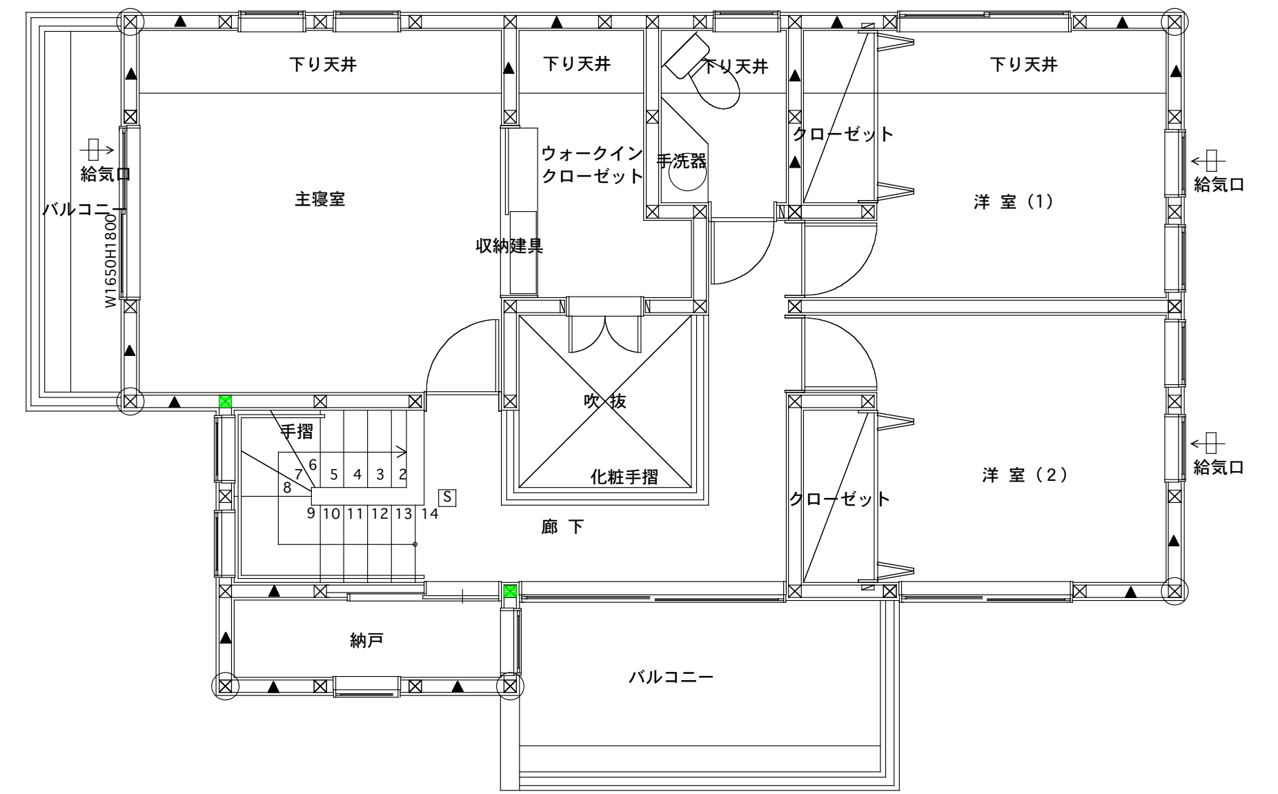
2階平面詳細図
